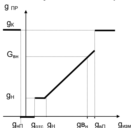
Рисунок 2.5 – Преобразование измеренных значений массового расхода
