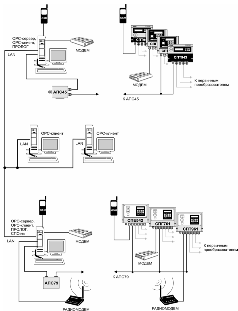
Рисунок 2.2 – Система информационного обеспечения учета энергоресурсов
